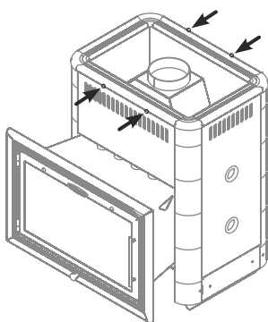
Рисунок 5. Демонтаж рамки конвектора печи «Витрувия»
