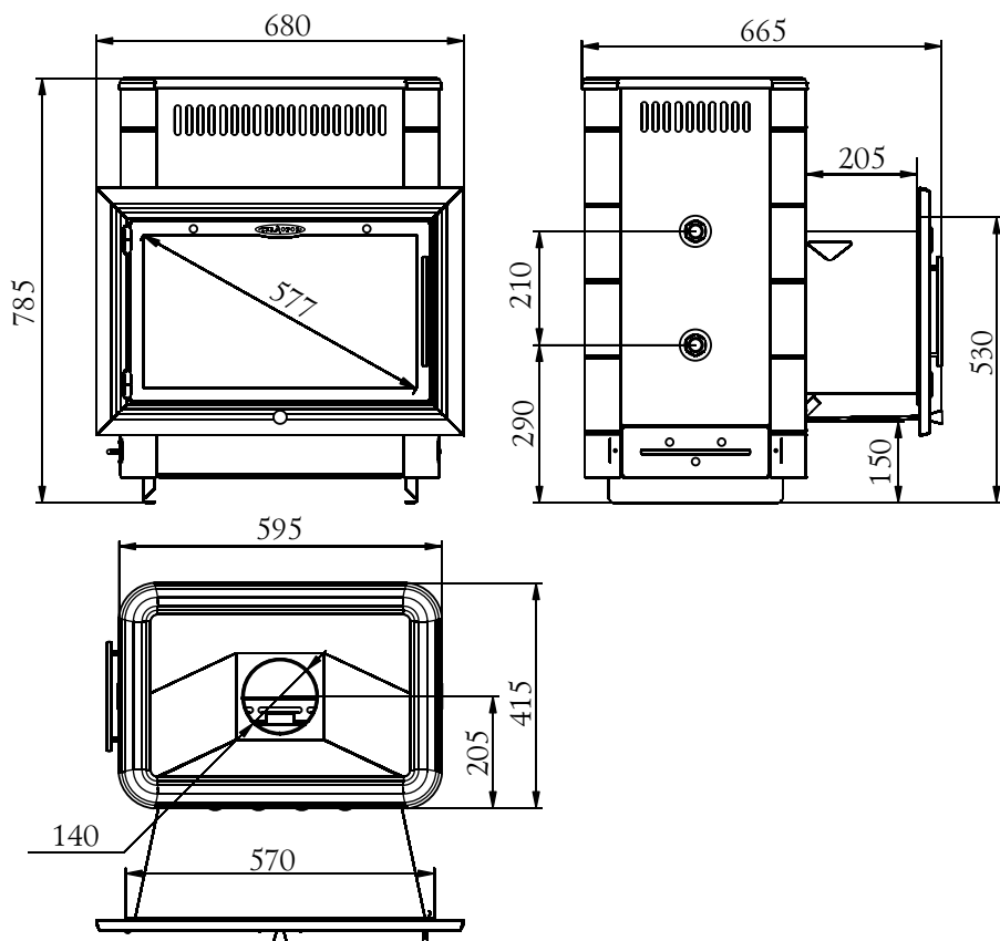
Рисунок 1. Габаритные размеры печи «Витрувия»
