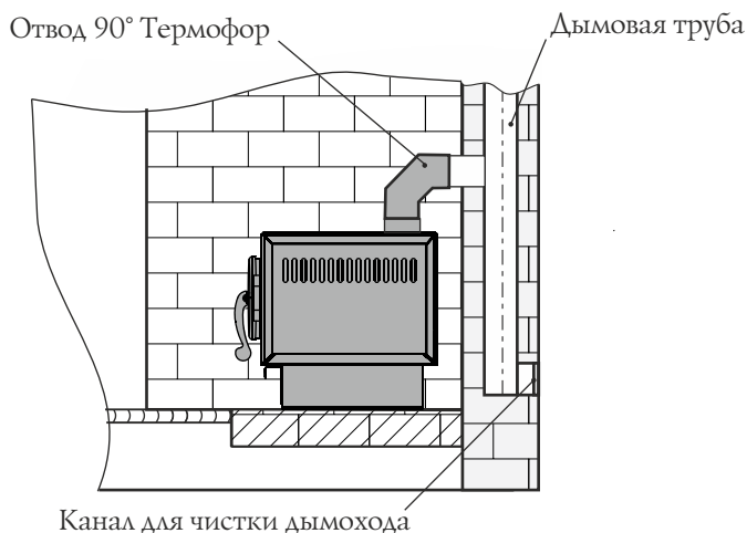
Рисунок 5. Схема присоединения печи к стационарному дымоходу из кирпича в помещении из негорючего материала.
